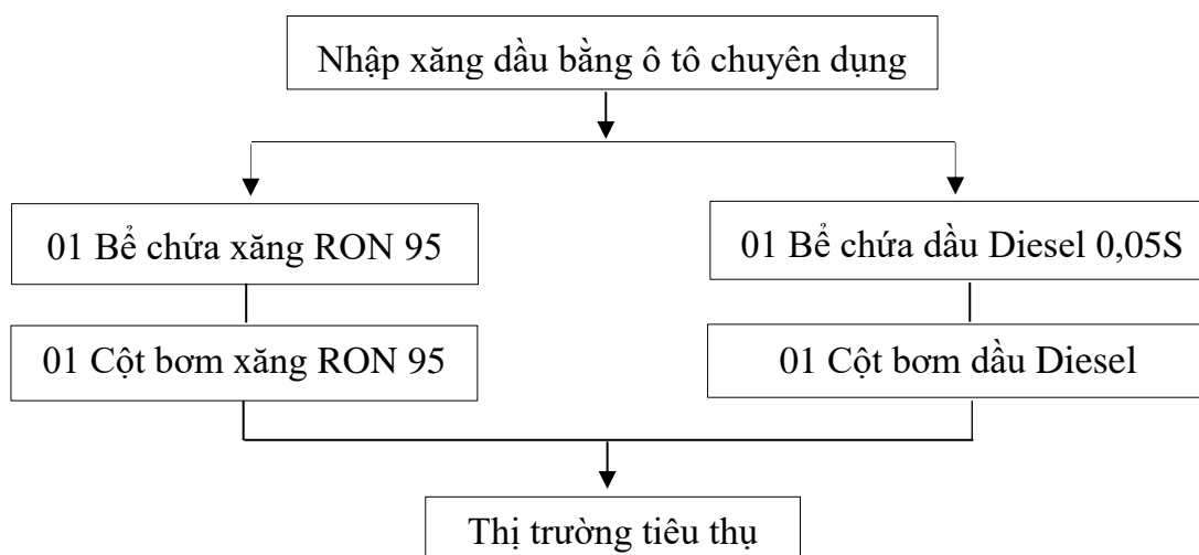
Hình 1.1. Sơ đồ quy trình công nghệ xuất nhập xăng dầu của Cửa hàng
